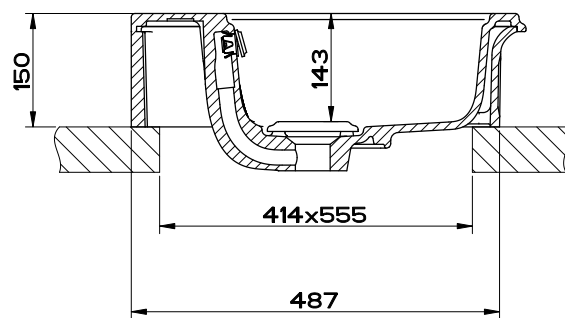
SEZIONE B-B
