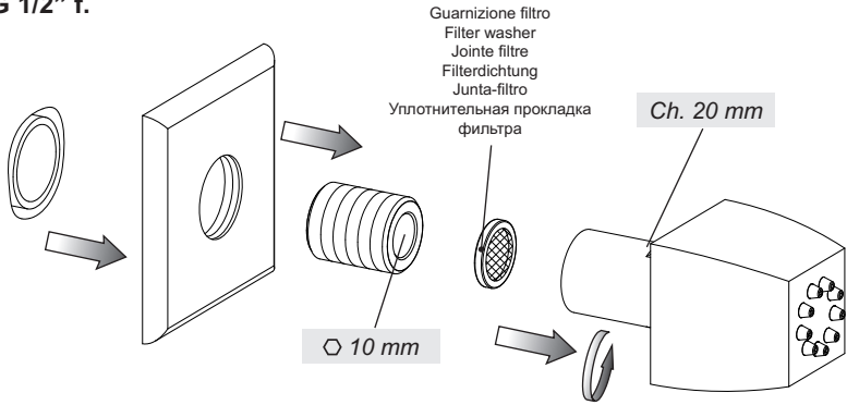
Fig. 5 - G 1/2" f.
