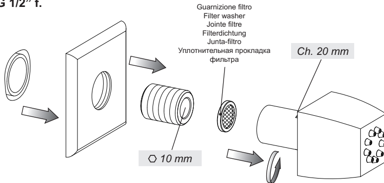
Fig. 8 - G 1/2" f.
