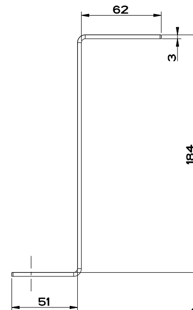
DETTAGLIO A SCALA 17:50
