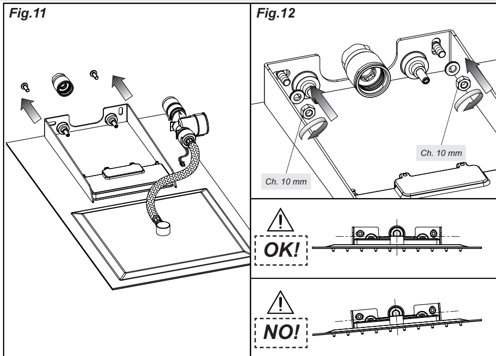
Fig. 11 - Avvicinare il soffione alla parete.
