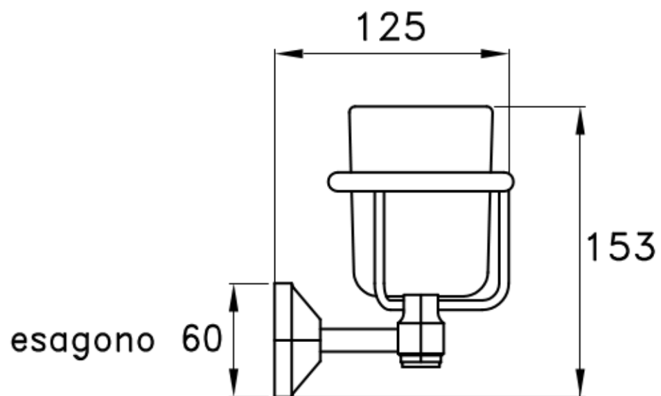
BICCHIERE VETRO
