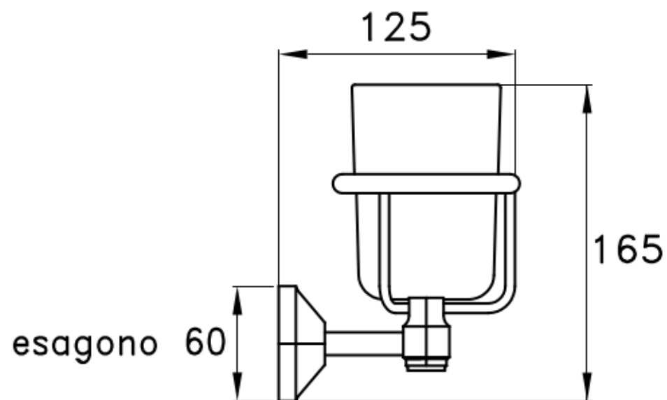
BICCHIERE CERAMICA
