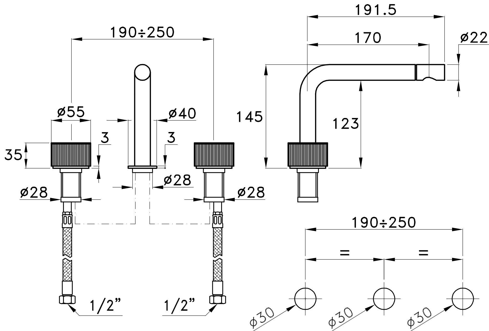
schema fori - modèle de trou hole pattern - patròn de agujero
